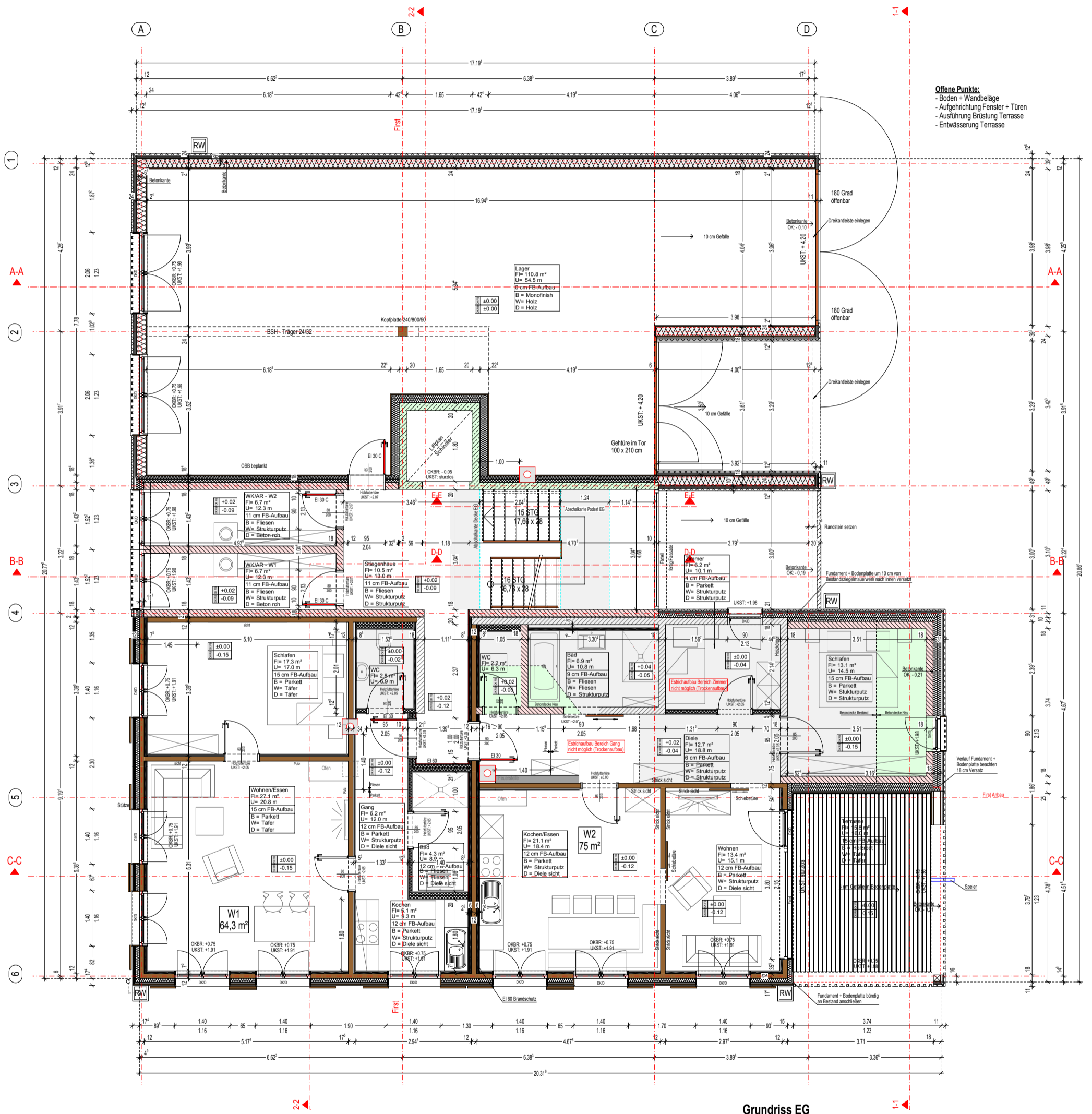
Grundriss EG
